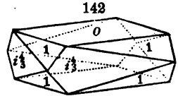
Wulfenite.
